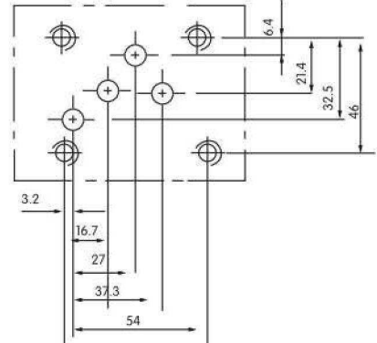
03系列安裝面 ISO4401-AC-05-4-A
