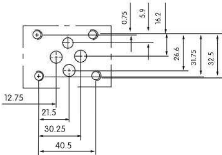
02系列安裝面 ISO4401-AB-03-4-A
