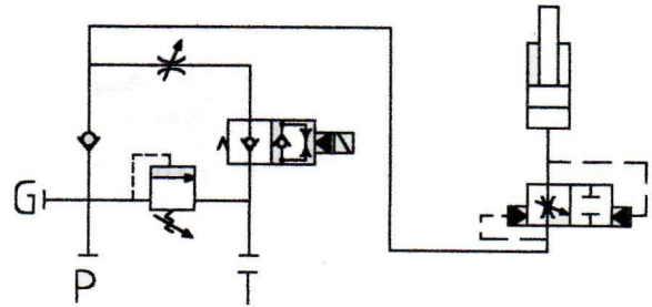
VF 系列防爆閥 油壓迴路圖
