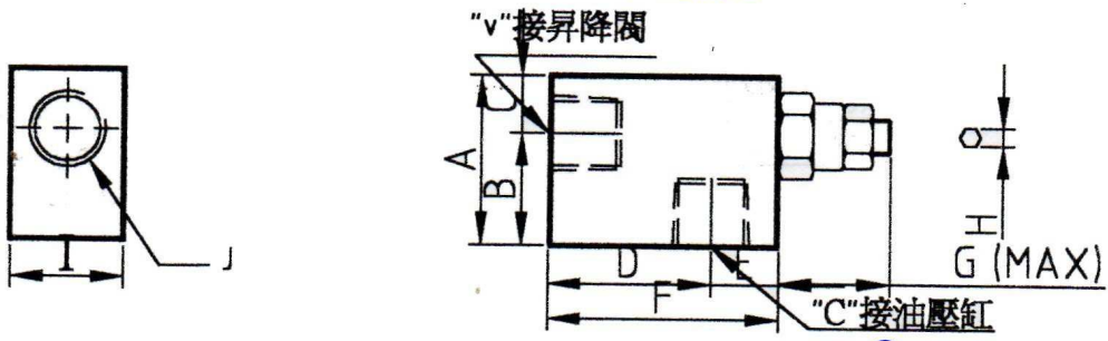
VF-30、80、120外形圖
