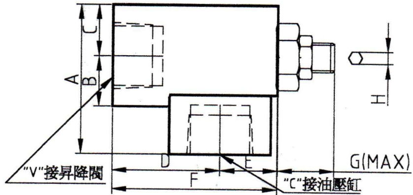
VF-160外形圖
